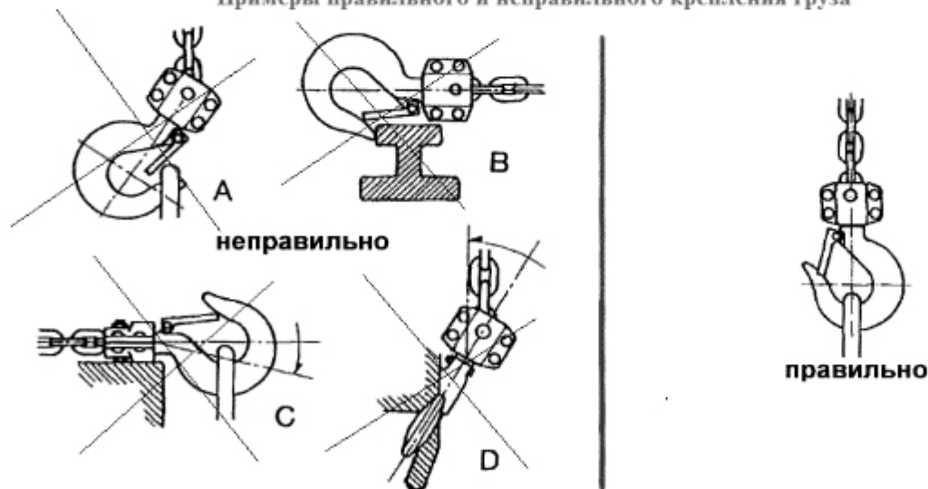
Примеры правильного и неправильного крепления груза
